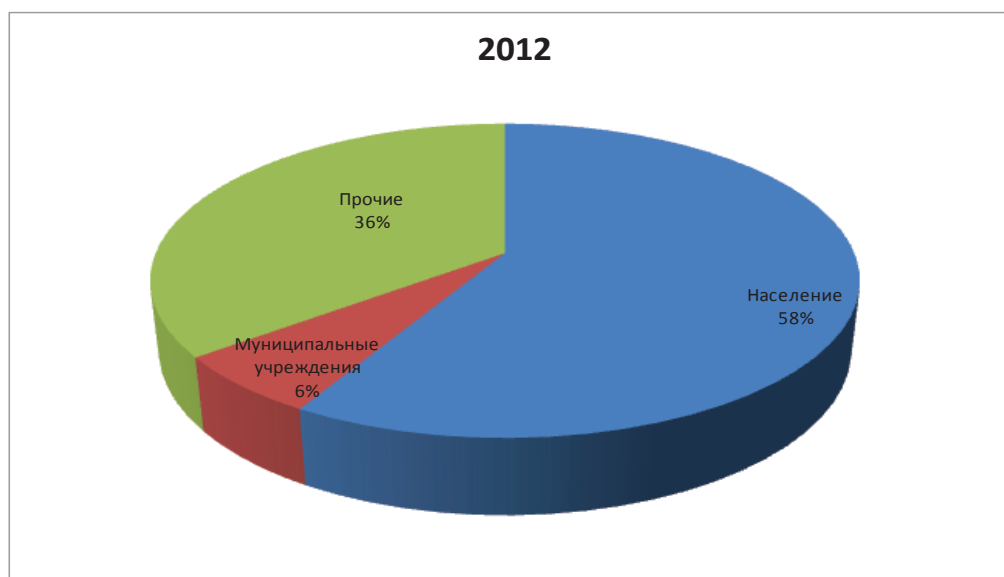
Рис. 2. Структура потребления тепловой энергии (Заречный)
